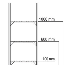
Abb. 15 Anordnung vordere Traverse Disposition des longerons avant Plaatsing dwarsbalk aan de voorzijde Arrangement of the front cross-arm
