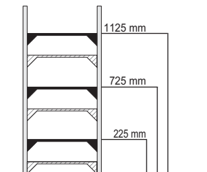
Anordnung hintere Traverse Disposition des longerons arrière Plaatsing dwarsbalk aan de achterzijde Arrangement of the rear cross-arm
